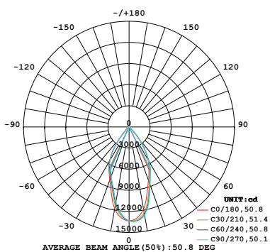
3L-25L medium 60°
